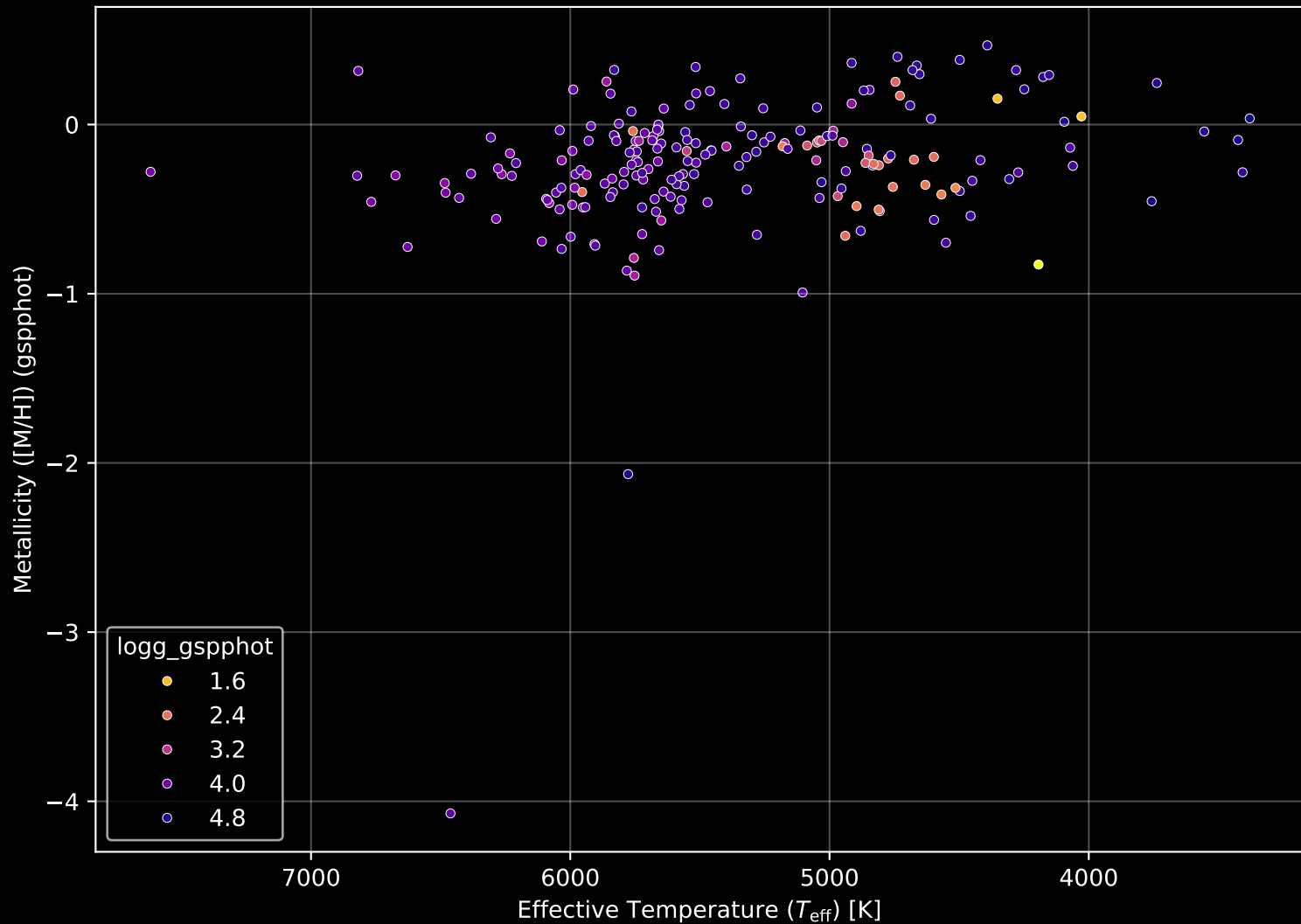
APOGEE DR17 Field: [273-41-O_TESS] Stellar Population Parameters (n= 206)
